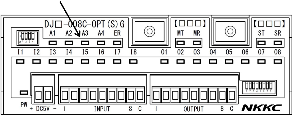
アドレス用 LED (A1, A2, A3, A4)
