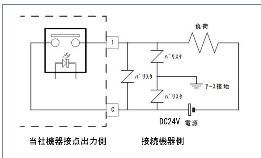
【図 9】 バリスタ設置例
