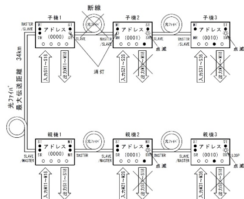
LOOP 回線が無い場合(システムダウンしている状態)
