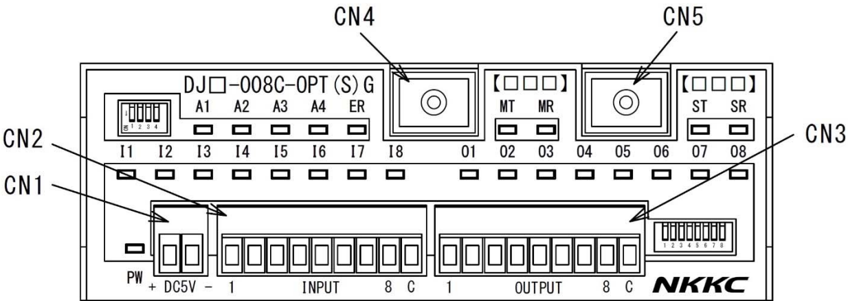
CN4 : 光ポート 親機 (LOOP/MASTER) / 子機 (MASTER/SLAVE)
