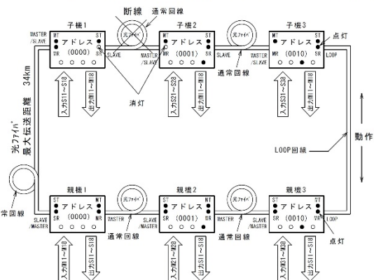
LOOP 回線がある場合(冗長機能が動作している場合状態)
