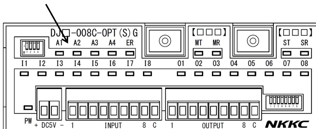
アドレス設定用スイッチ
