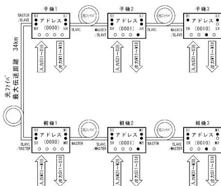
LOOP 回線が無い場合(正しく接続されている状態)
