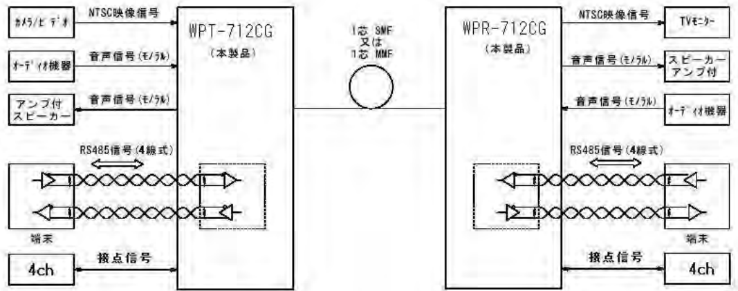
図3 接続構成
