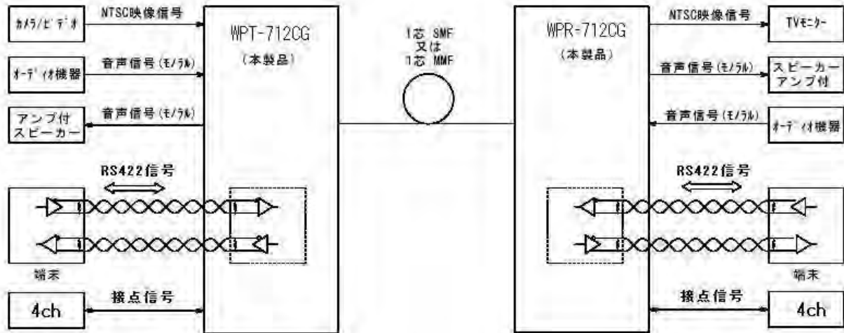
図5 接続構成
