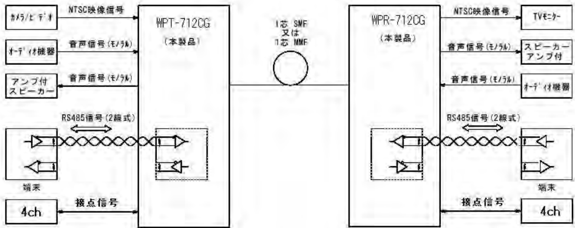
図1 接続構成
