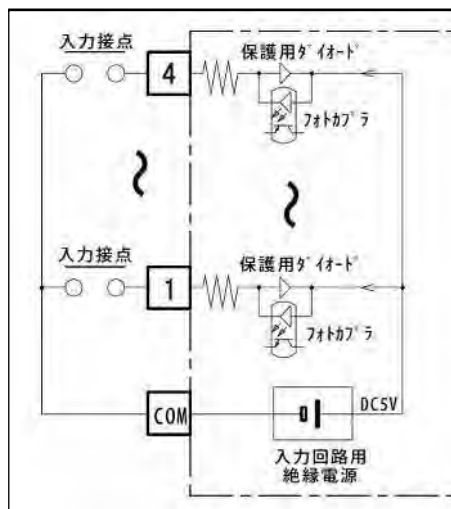
入力構成
