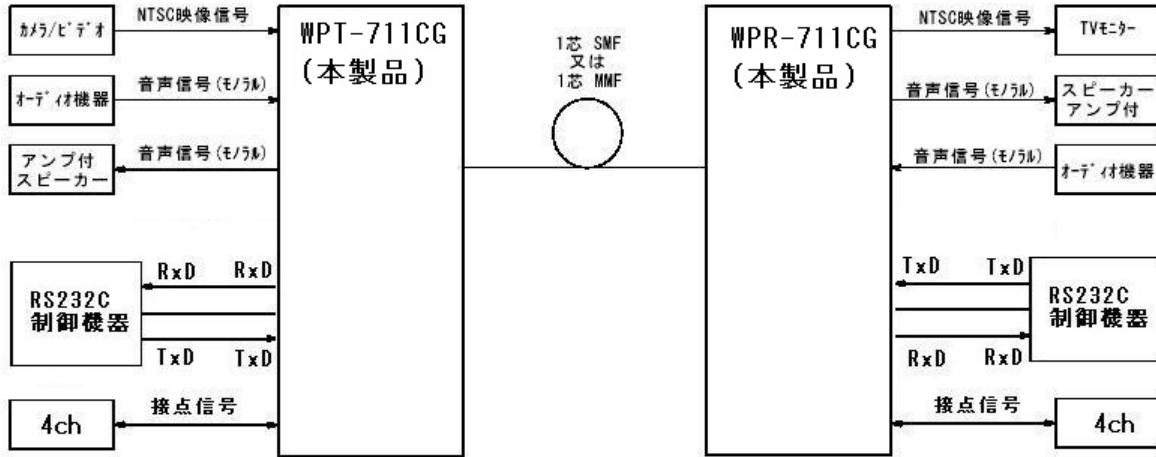
図1 接続構成
