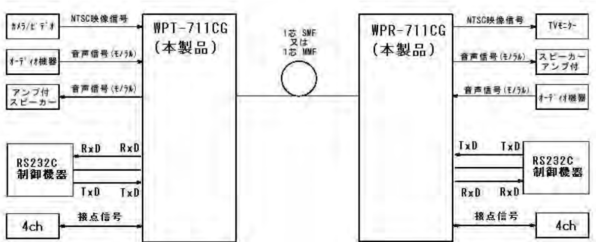
図1 接続構成
