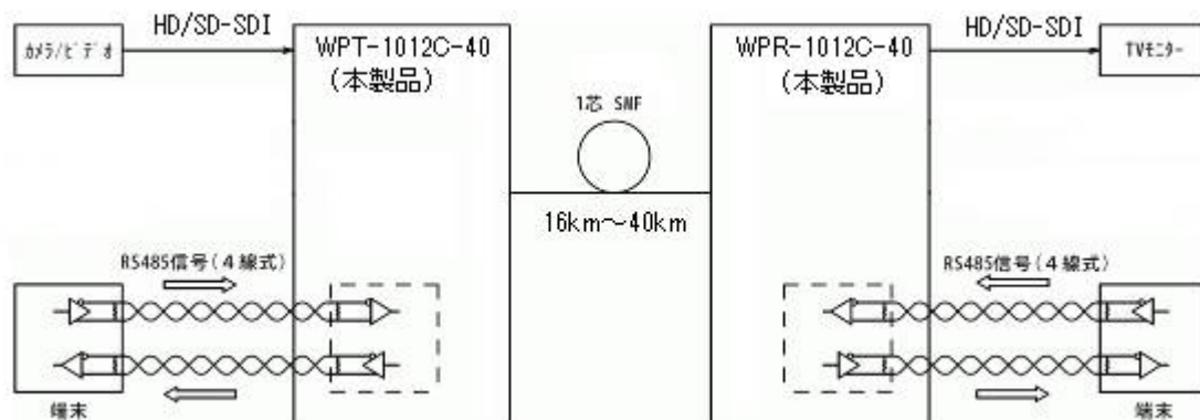
図1 接続構成
