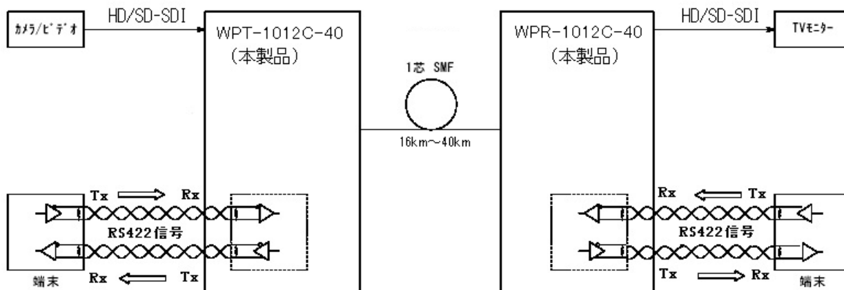
図 1 接続構成
