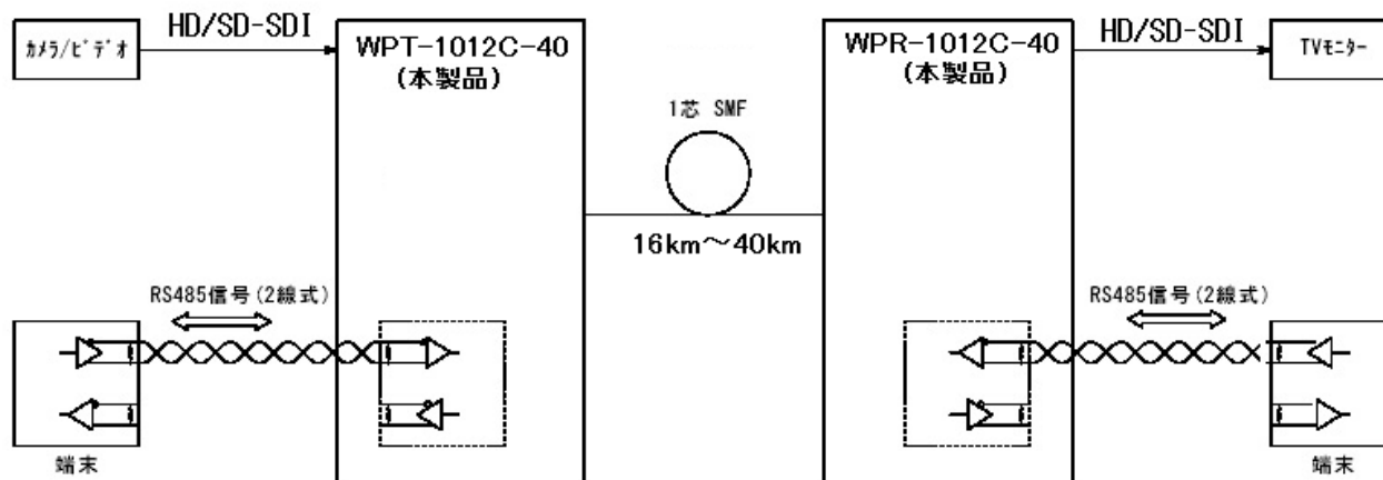
図1 接続構成
