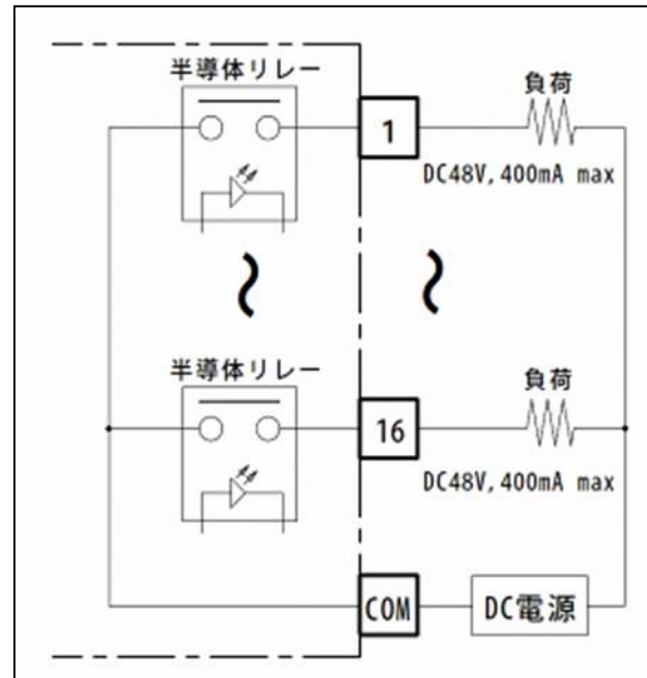
出力構成
