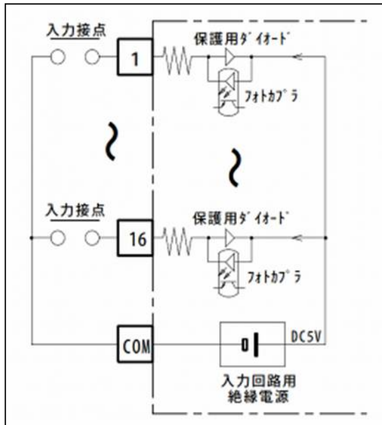
入力構成
