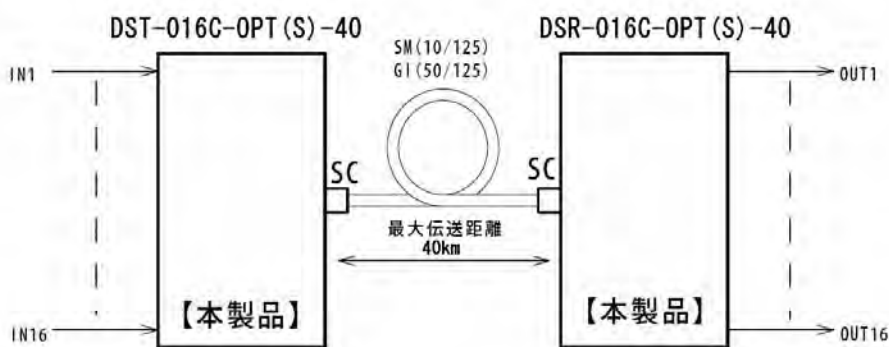
接続構成
