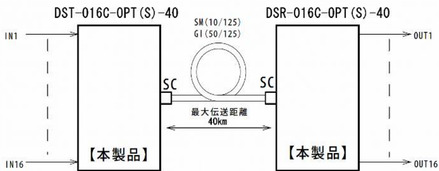
接続構成
