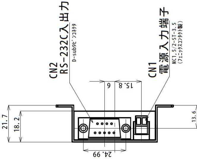
CN1: 電源入力端子
