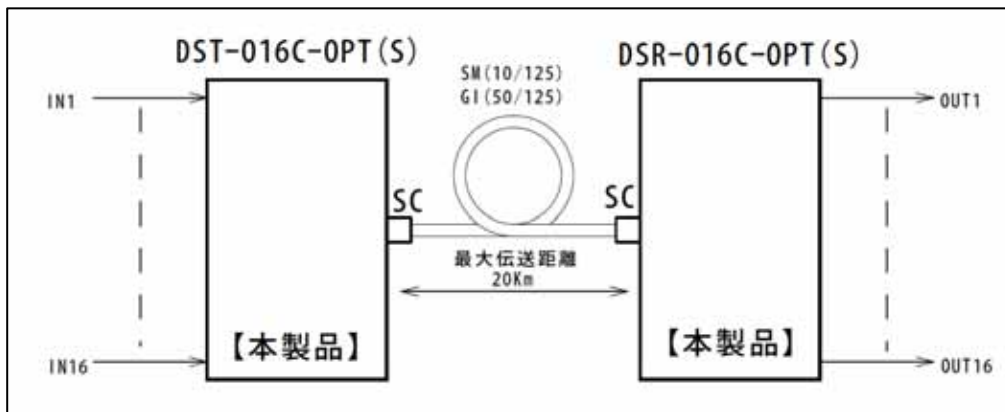
接続構成
