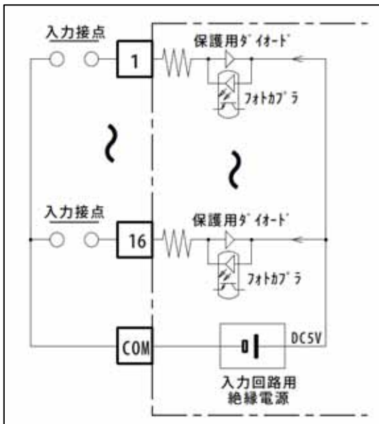
入力構成
