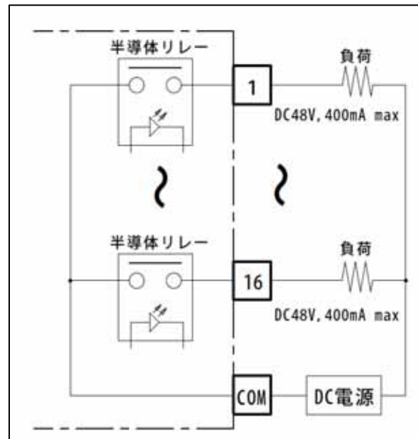
出力構成
