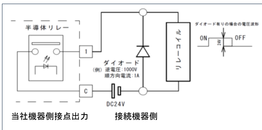
【図 2】ダイオード有り時の接続例
